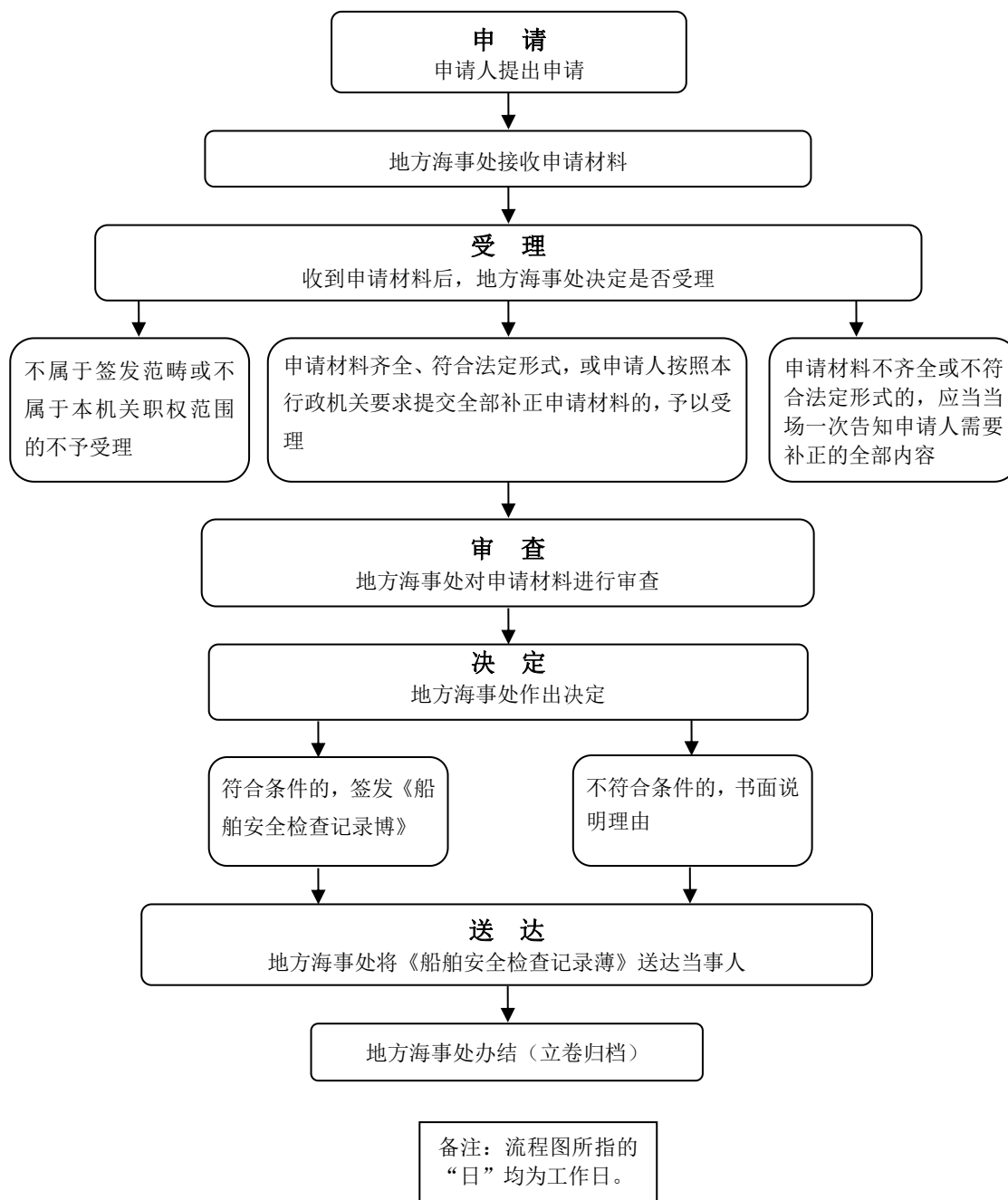
船舶《船舶安全检查记录簿》核发流程图
