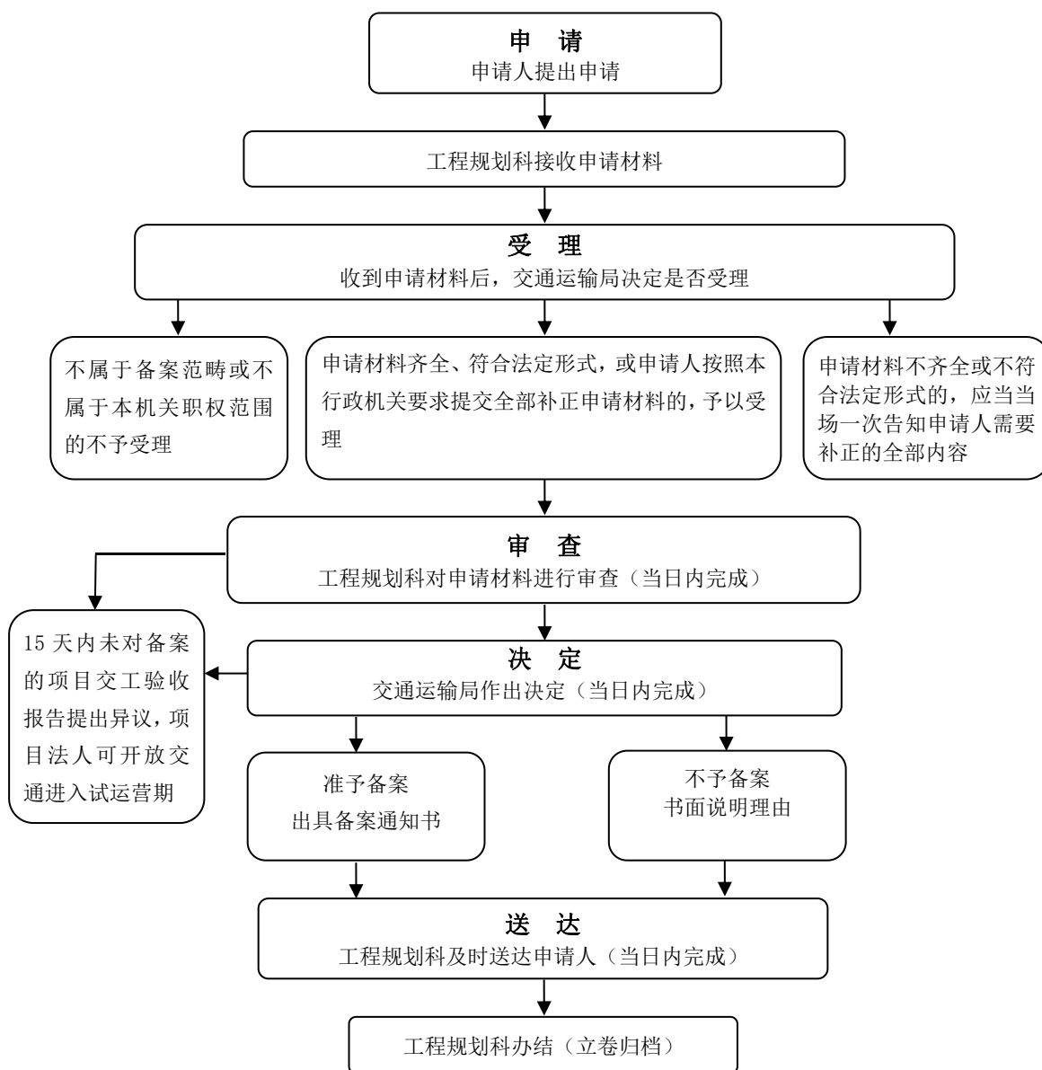
乡道、村道建设项目交工验收备案流程图
